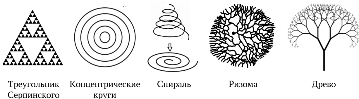
Рис. 11. Фрактальные модели
